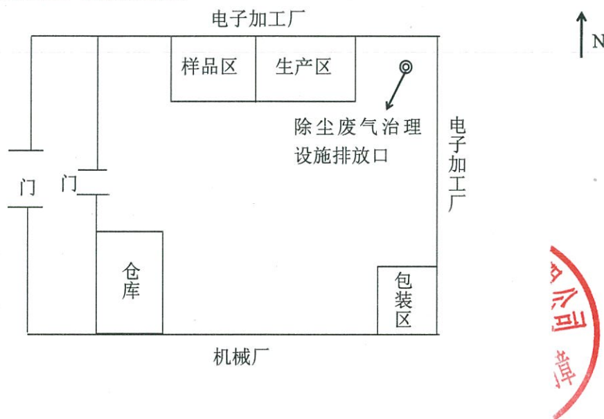
固定污染源有组织排放废气测点示意图
